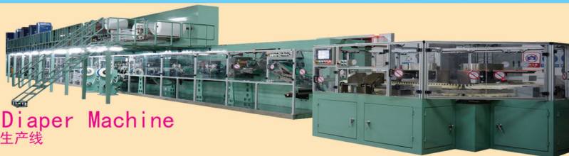
Baby Diaper Machine 婴儿纸尿裤生产线
